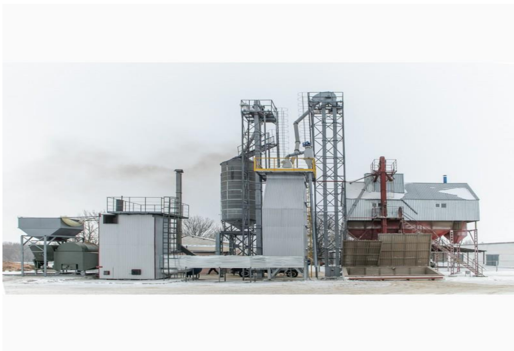
Рисунок 1 - шахтная зерносушилка (фото из интернета). Энергетические затраты в зависимости от марки – от 36,6 до 80 кВт
